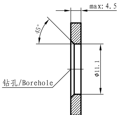
钻孔安装
